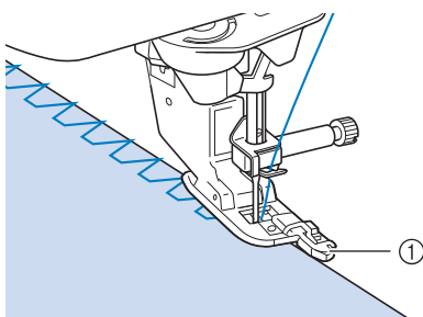
① Направляющая
