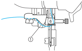
① Желобок нитенаправителя
