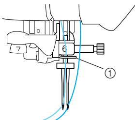
① Нитенаправитель игловодителя
