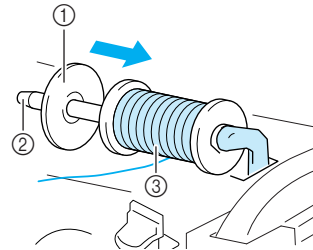
① Дополнительный стержень для катушки ② Колпачок катушки ③ Катушка с нитью
