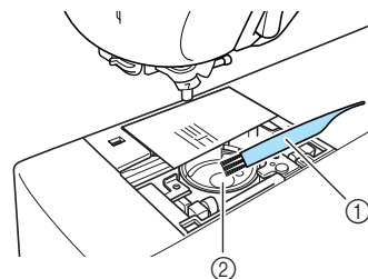
① Щеточка для очистки ② Челнок
