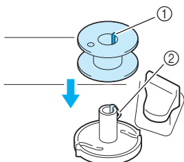
① Желобок на шпульнике ② Пружина вала устройства намотки шпульки
