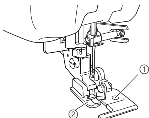
① Направляющая пластина (нижний нож) ② Прижимная лапка
