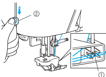
① Крючок ② Рычажок нитевдевателя
