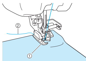
① Прижимная лапка ② Верхняя нить
