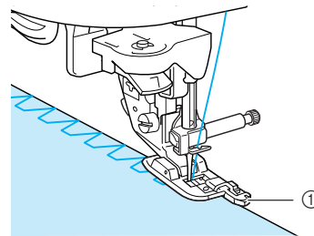
① Направляющая прижимной лапки
