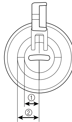
① 6,4 мм (около 1/4 дюйма) ② 9,5 мм (около 3/8 дюйма)
