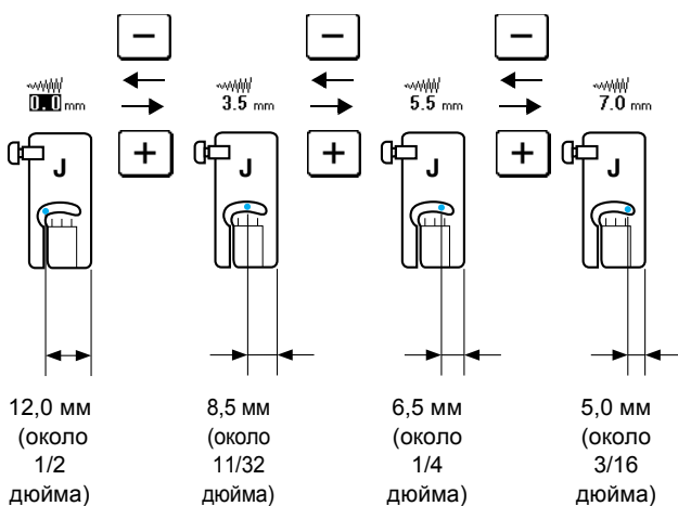
① Ширина строчки
